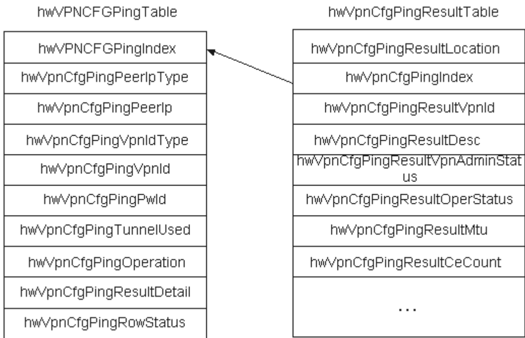
图 137-1 探测表与探测结果表的表间关系图
